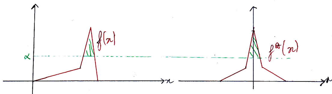
FIGURE 1.1 – Symétrisation d'un ensemble
